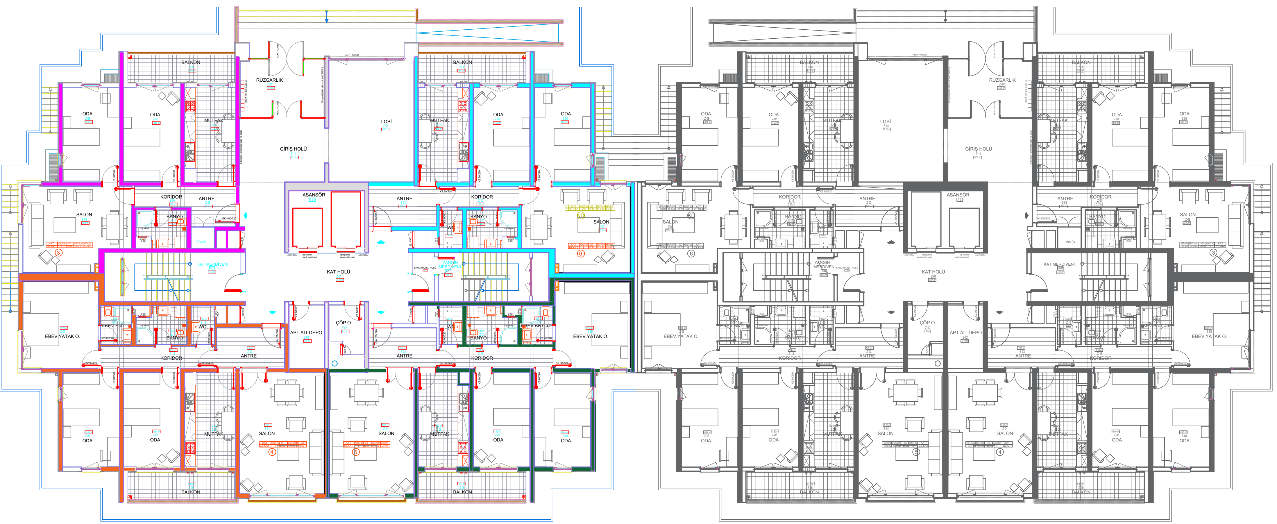
ANKARA SİNCAN SARAYCIK MAHALLESİ G.Ö.B. KENTSEL DÖNÜŞÜM PROJESİ SC TİP BLOK ZEMİN KAT PLANI
